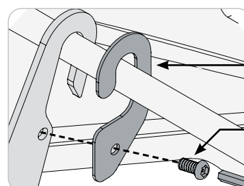
Panelock™ Hook
